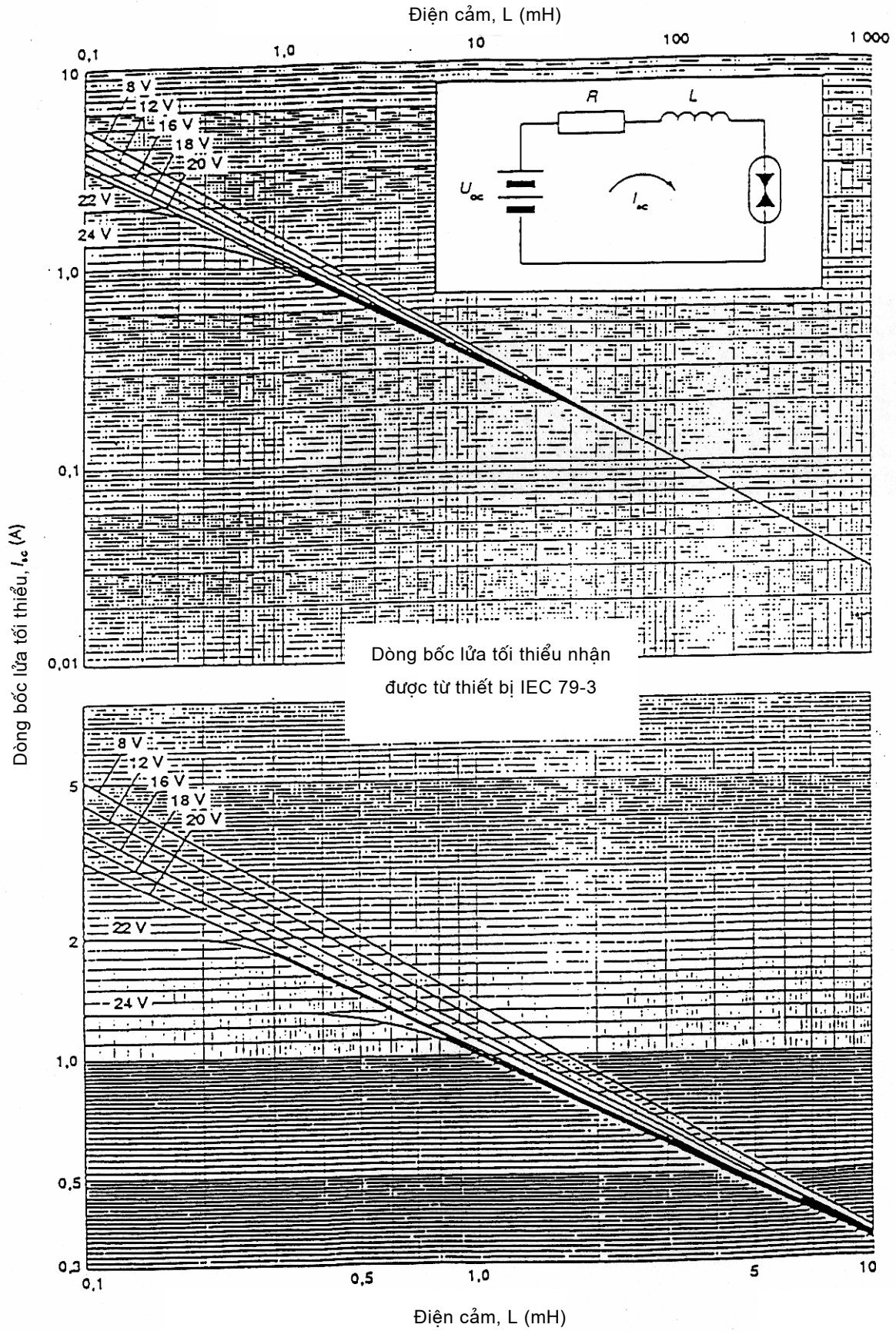
Hình C.4 - Mạch điện áp thấp
