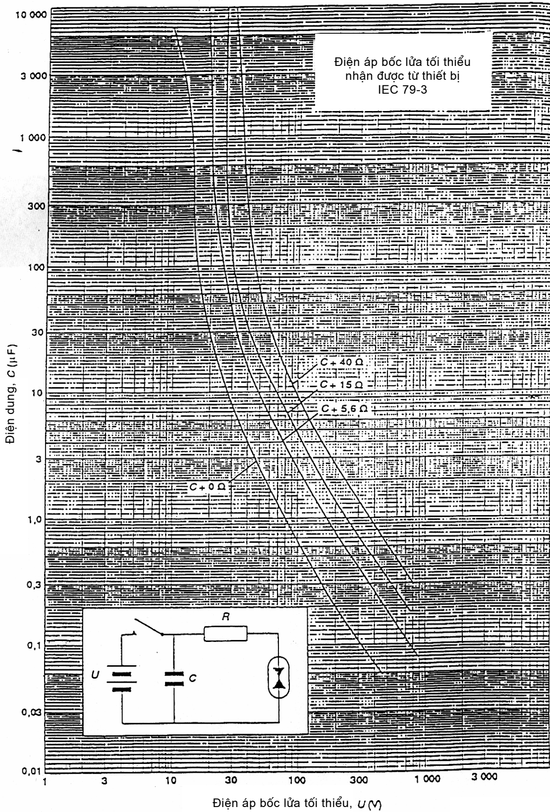
Hình C.2 - Mạch điện dung
