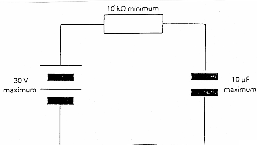
Hình C.5 - Mạch thuần dung
