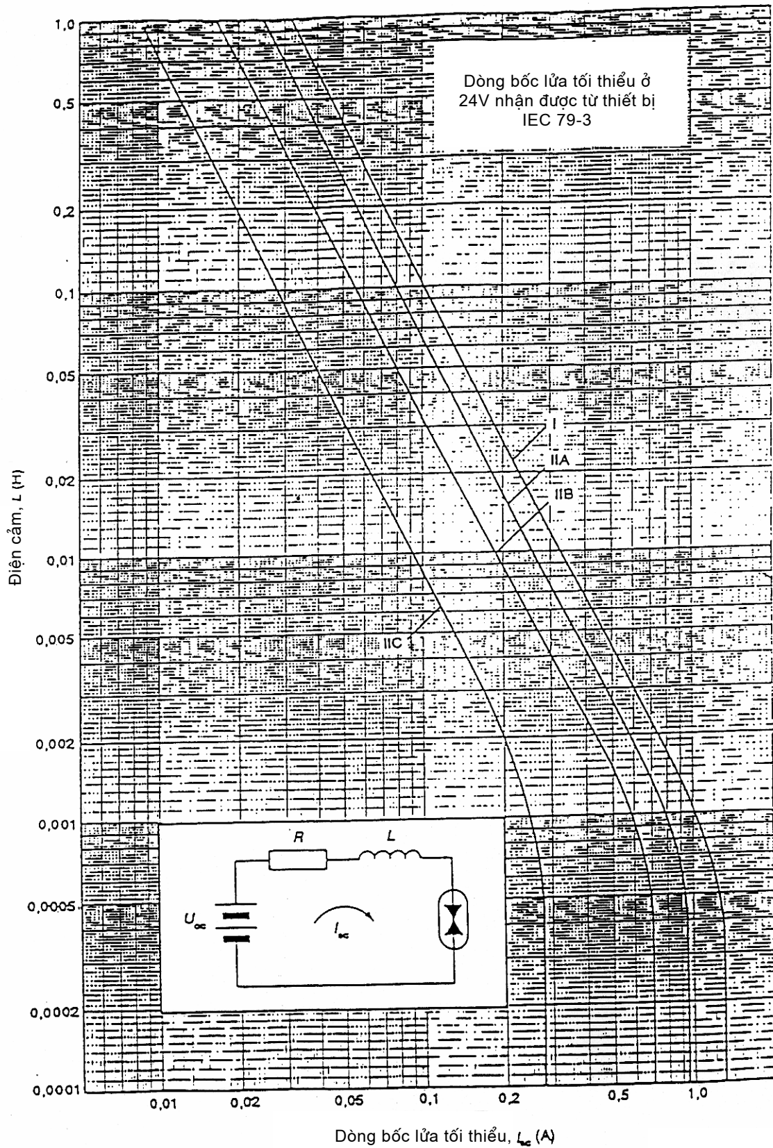
Hình C.3 - Mạch điện cảm
