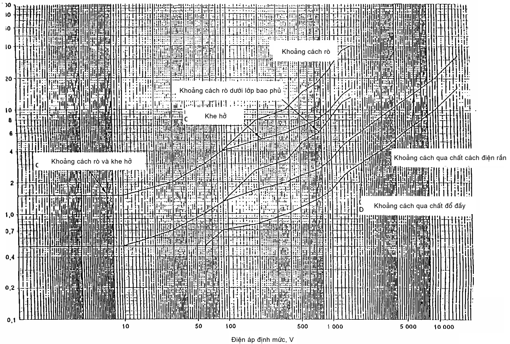
Hình A.5 - Các giá trị đồ thị từ bảng 4 phục vụ cho việc nội suy. Tất cả kích thước của các đường tính bằng mm
