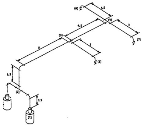
Hình 4 – Hệ thống không cân bằng điển hình
