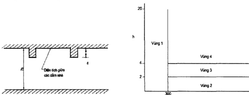
Hình 4 - Yêu cầu thiết kế cho các đầu báo cháy khói kiểu điểm và các hệ thống đầu báo cháy khói kiểu hút trong các cấu trúc nhà có dầm
