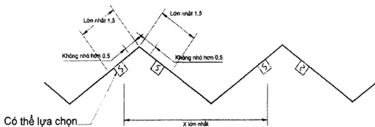
(c) Bề mặt dốc như nhau
