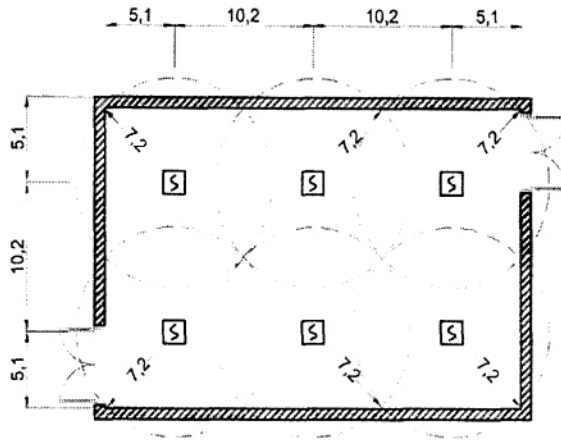
Hình 2 - Khoảng cách lớn nhất giữa các đầu báo cháy lắp đặt trên bề mặt bằng trần phẳng
