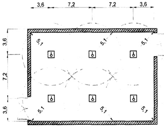
Hình 7 - Khoảng cách lớn nhất giữa các đầu báo cháy nhiệt trên bề mặt bằng phẳng
