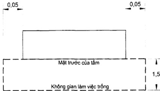
Hình 10 - Khoảng hở nhỏ nhất đến kết cấu bao che khu vực bảo vệ
