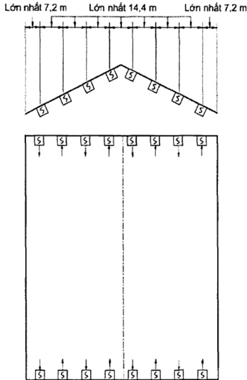
Hình 5 - Ví dụ về các vị trí của đầu báo cháy khói tia chiếu
