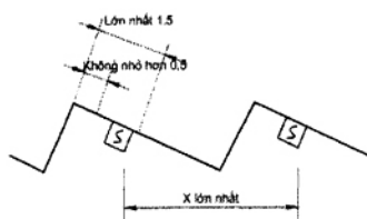
(a) Bề mặt dốc khác nhau
