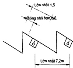
(b) Trần, mái hoặc bề mặt dạng răng cưa
